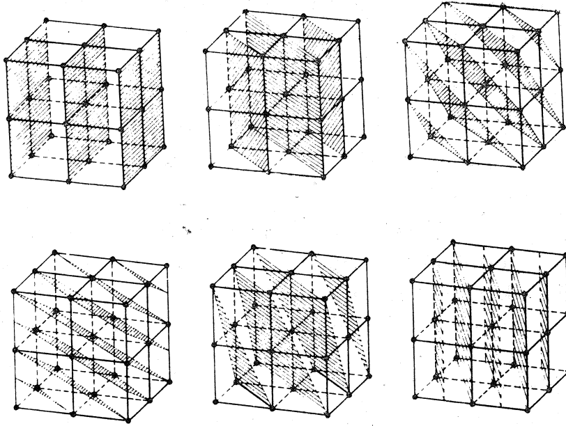
Şek. 1 - Kübisal sistemde özdeş ağ yüzeylerin örnekleri.
