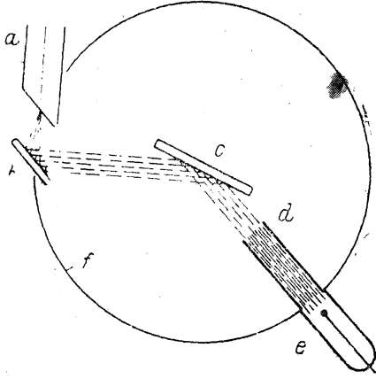
Şek. 5 - Röntgen flüoresans analizde ışın yolu.
