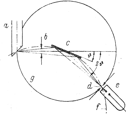
Şek* 4 - Yansıtma ile röntgen analizinde ışın yolu»
