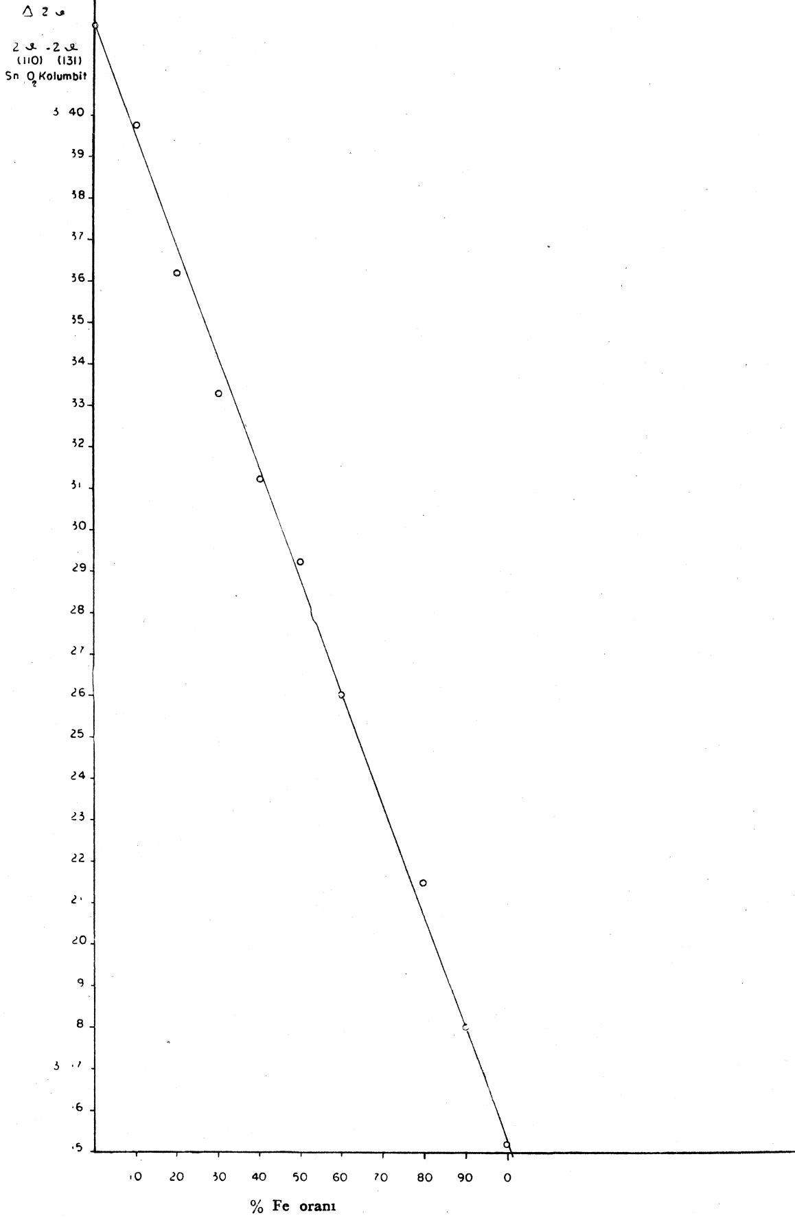
Şek. 2 - Kolumbitlerdeki Fe oranına göre 2 \theta nın değışimi. (131)
