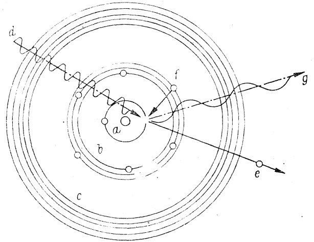
sek. 3 - Niels Bohr atom 'modeli ve röntgen spektrumunun oluşumu.
